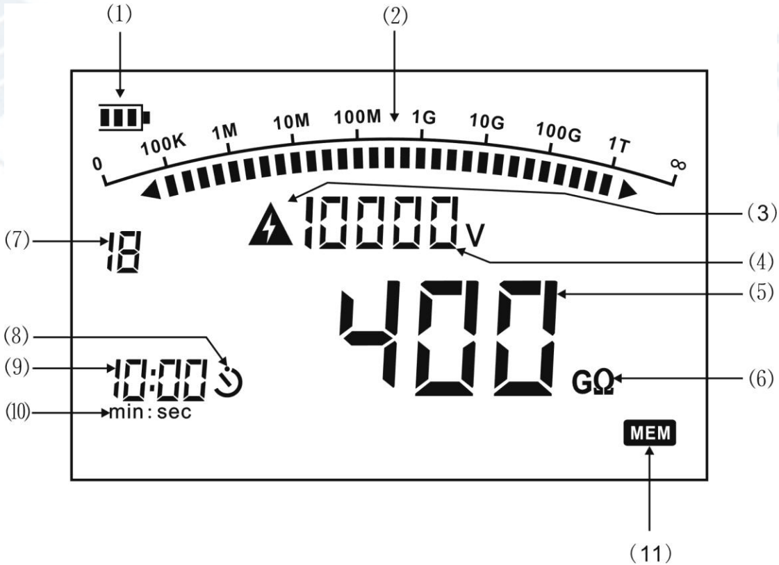
图2： TE8675液晶显示内容
