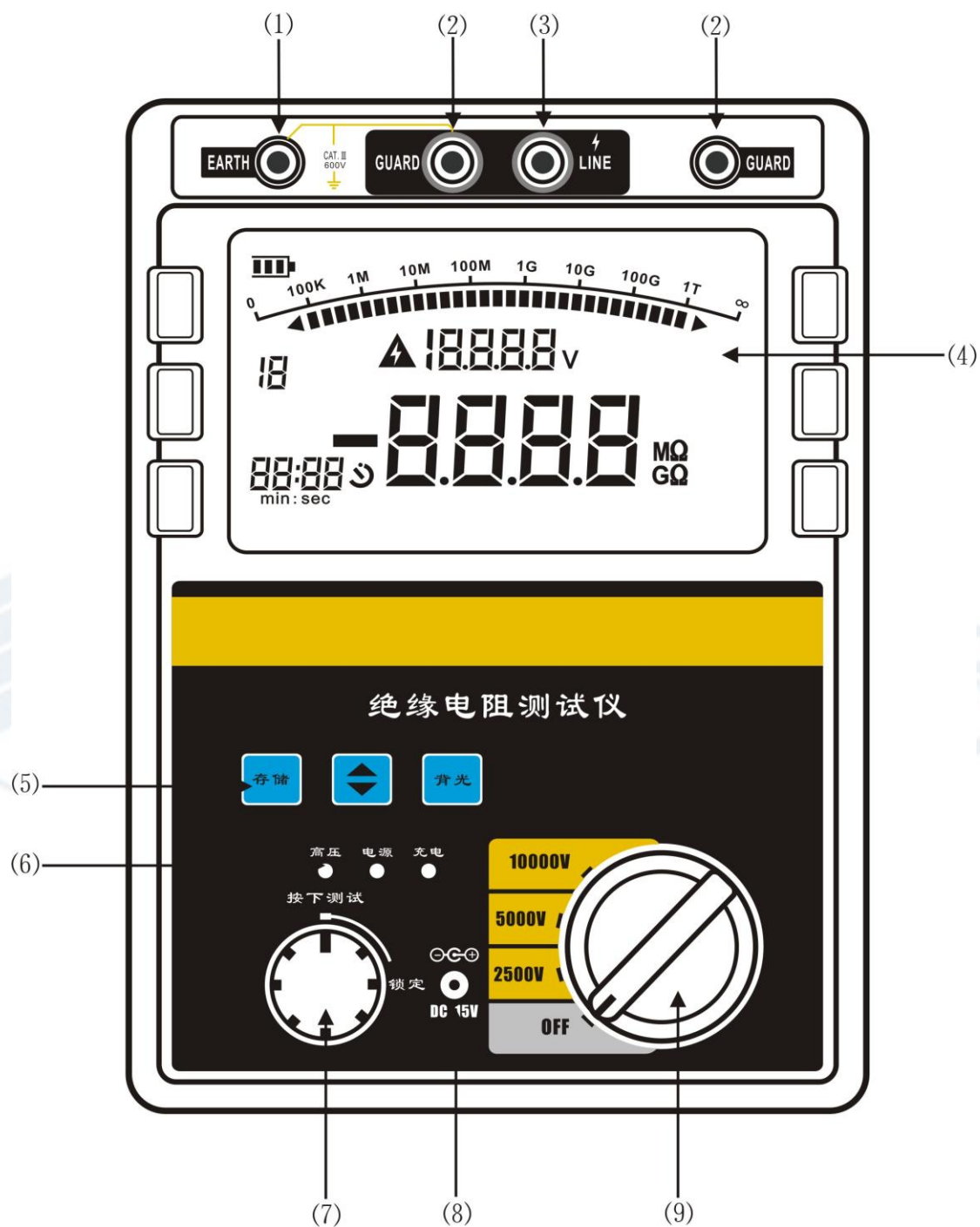
图 1：TE8675 面板结构说明
