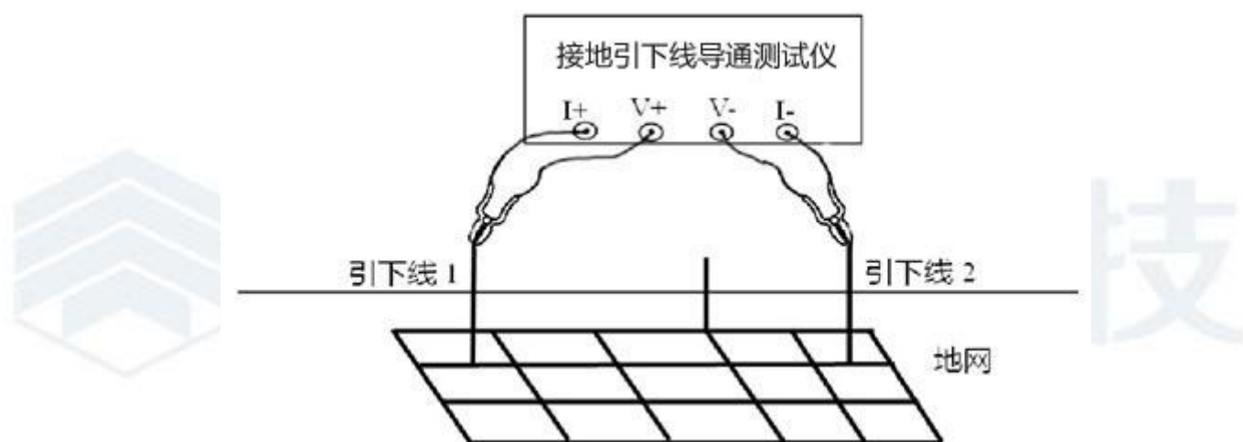
图三 四端子接线图
