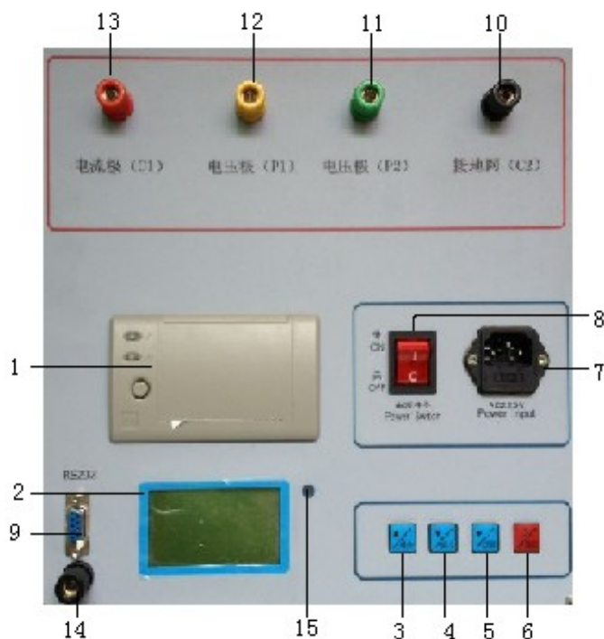
面板示意图
