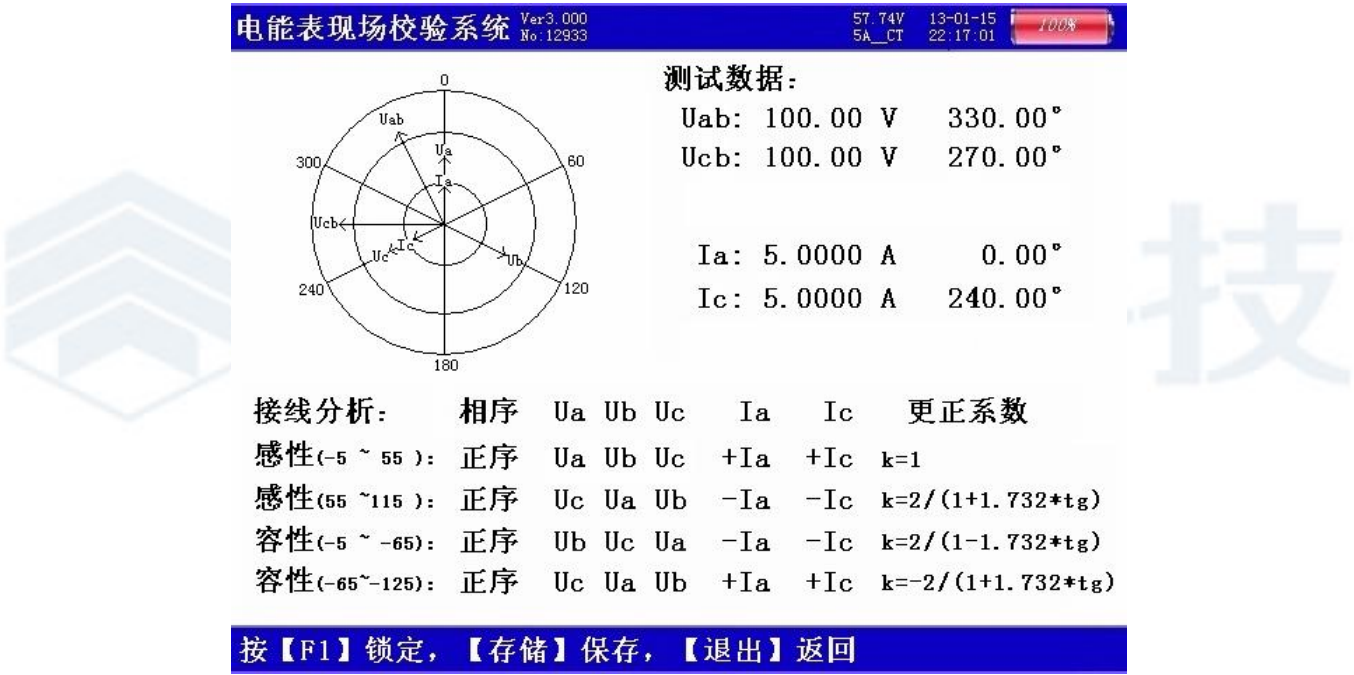
图九、矢量分析屏—三相三线
