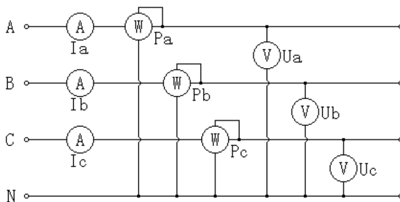
图十七、三相四线计量原理图
