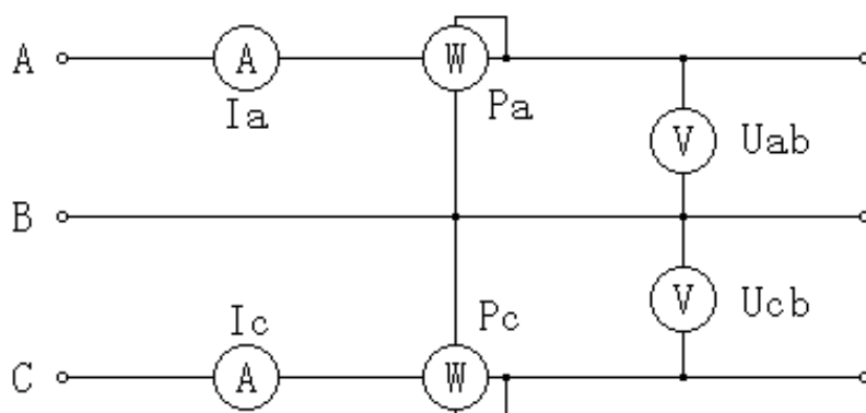
图十六、三相三线计量原理图
